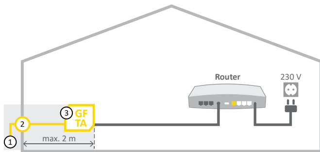
Abbildung 1: Beschreibung Glasfaser-Hausanschluss
